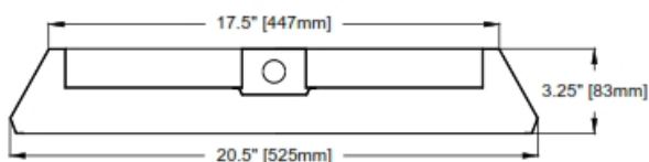
S HB-20 End
