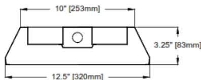
S HB-12 End
