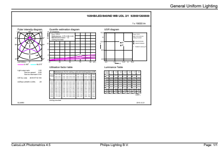
NAM Highbay 165W-400W 4000K 120D E39X UDL
